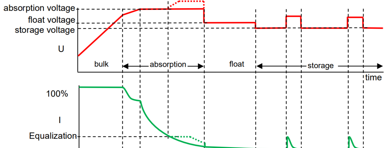
Bild 3 Spänning och ström under olika lägen i batteriladdning.
