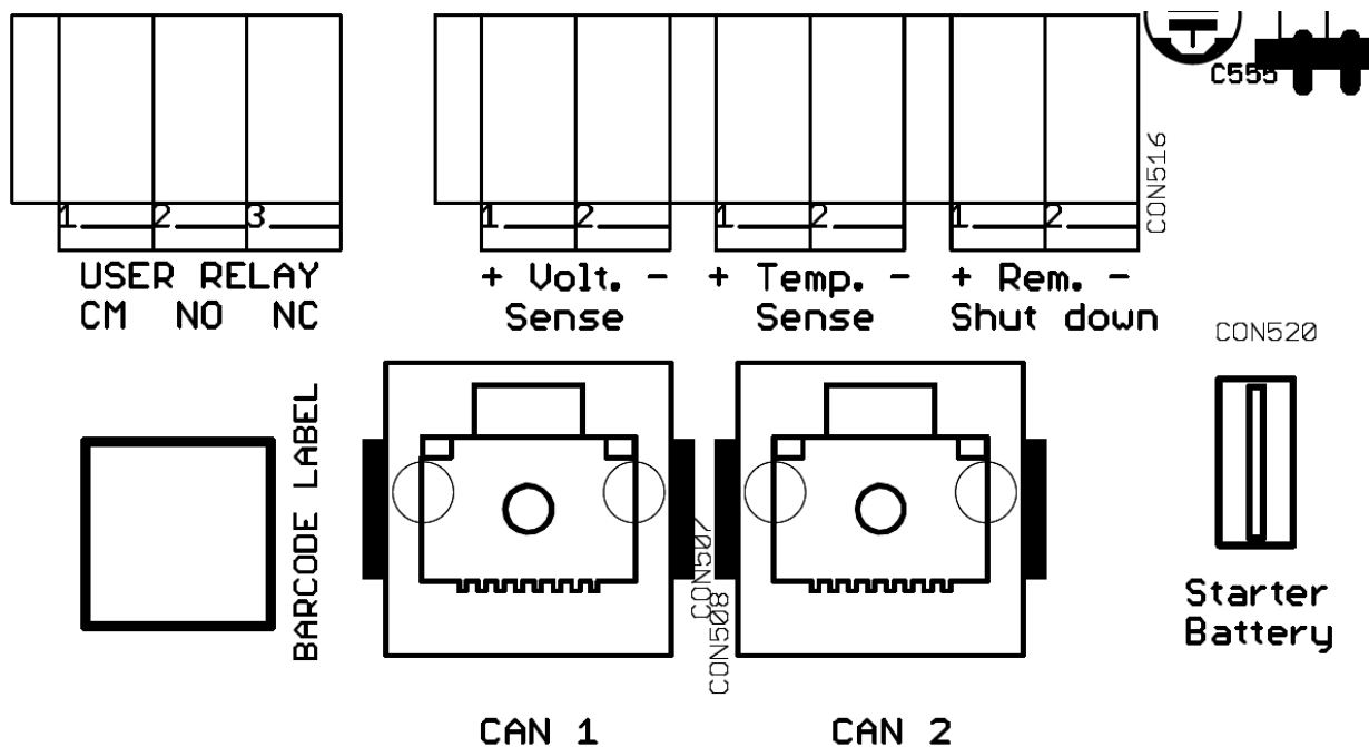
Bild 1 Kontakter för extern spänning-/temperaturkontroll, fjärr- avstängning, VE.Can-bus och startbatteri.
