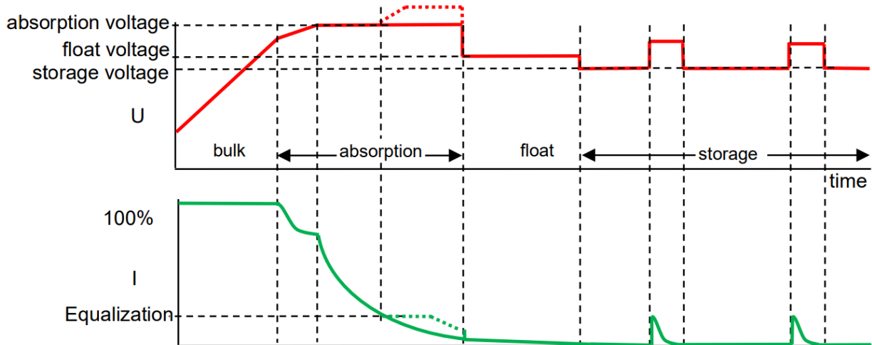
Figura 3 La tensión y la corriente durante distintas fases de la carga de la batería.
