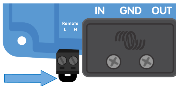
Fjärrstyrd av/på-kontakt med metallögla
