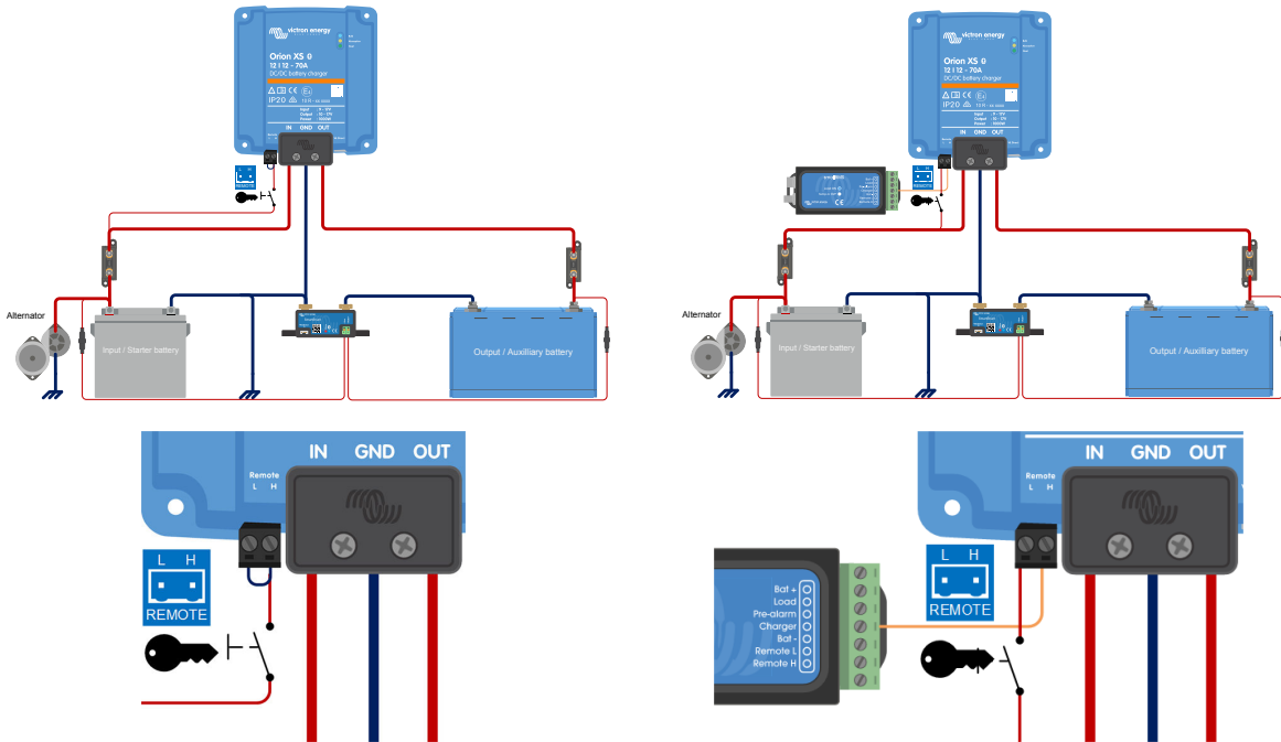
Anslutningsdiagram för att förbigå avkänning av motorfrånkoppling
