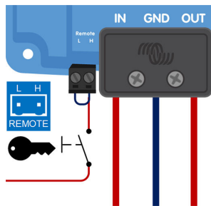
Diagrama de conexión de la anulación de la detección del apagado del motor
