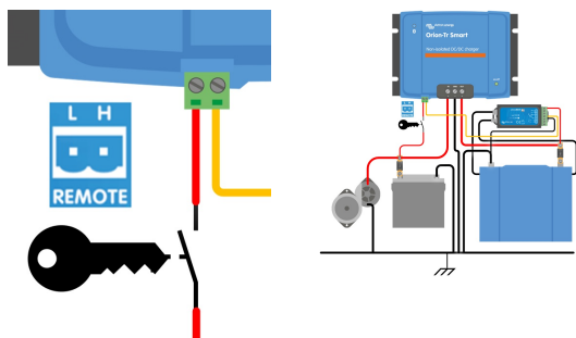
Figura 4: Schema delle connessioni dell'esclusione del rilevamento di arresto motore
