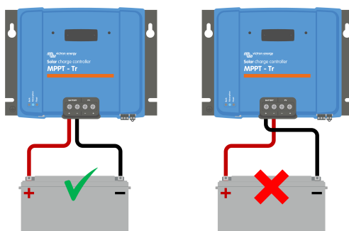
Voorbeelden van juiste en onjuiste (omgekeerde) accupolariteit.
