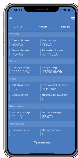
VictronConnect-app toont de historie van de accumonitor
