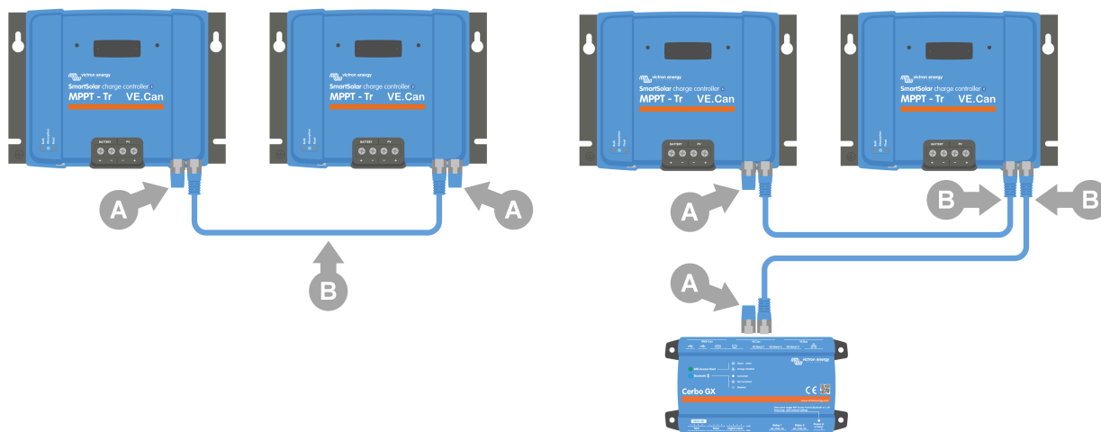
A: VE.Can-afsluiting - B: RJ45 UTP-kabel:
