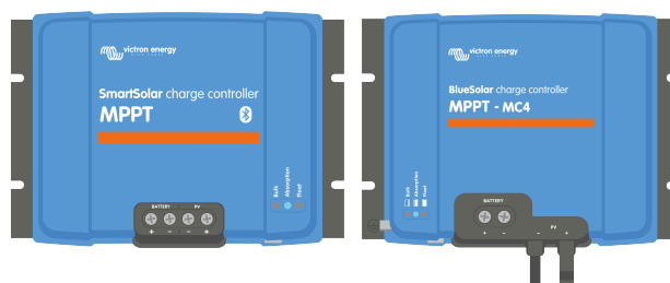
Van links naar rechts: Voorbeeld van zonneladers met schroefklemmen en MC4 PV-aansluitingen
