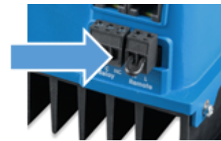
Fernbedienungsstecker mit Drahtschleife.
