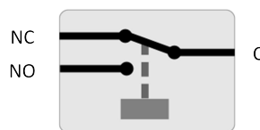
Configuration du relais (non alimenté)
