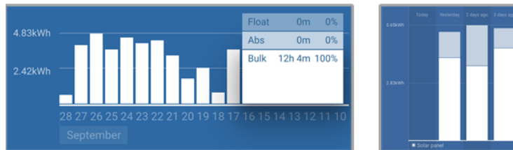
Vasen: Esimerkki järjestelmästä, joka on koko ajan päälataustilassa. Oikea: erittely lataustiloista - Järjestelmä on pää- ja absorptiolataustilassa.
