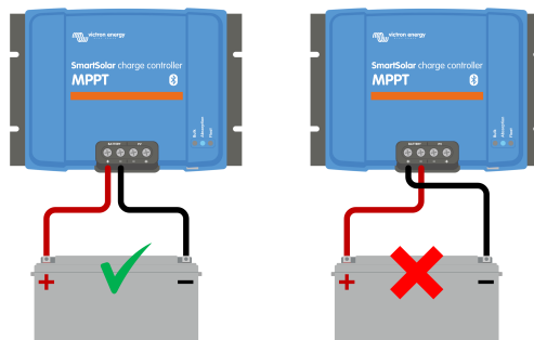
Esimerkkejä oikeasta ja väärästä (ristiin kytketystä) akun napaisuudesta.
