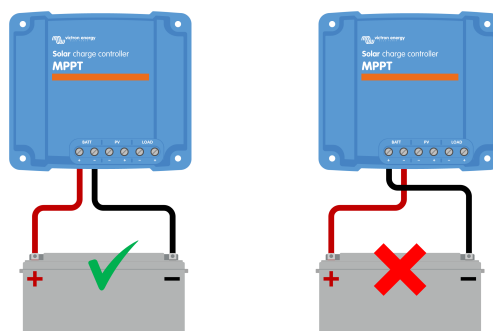
Exempel på korrekt och inkorrekt (omvänd) batteripolaritet.
