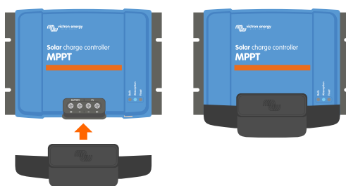
Exemplu încărcător solar cu MPPT WireBox
