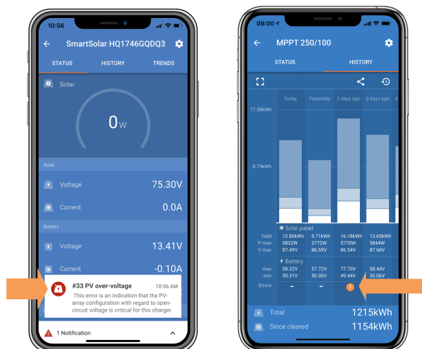
Visning i statusskärmen och historikskärmen av fel #33 i appen VictronConnect.
