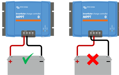
Exempel på korrekt och inkorrekt (omvänd) batteripolaritet.
