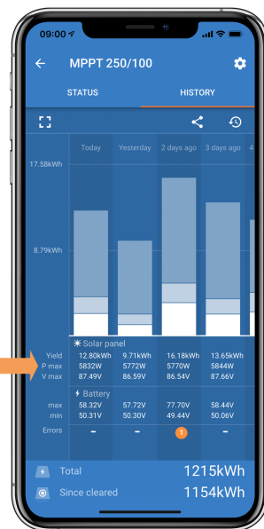
Avläsning av Pmax-historik i appen VictronConnect.
