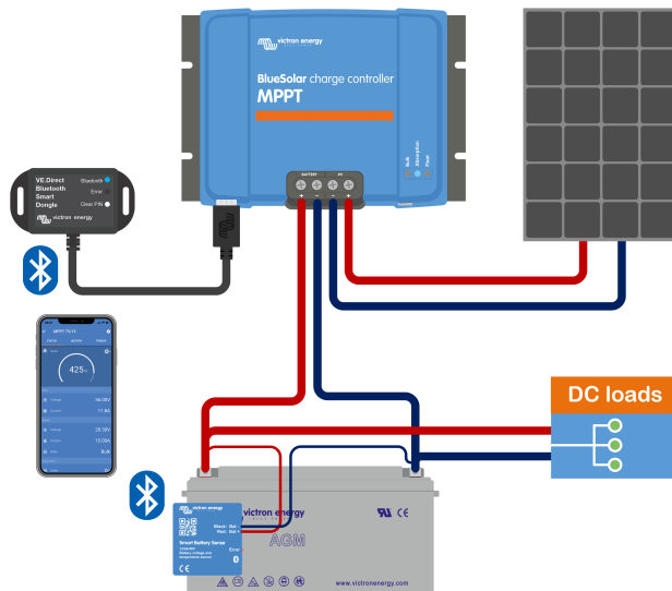
Beispiel für ein VE.Smart-Netzwerk aus einem Smart Battery Sense und einem Solarladegerät.
