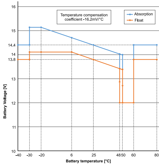
Temperaturkomparerat laddningsdiagram
