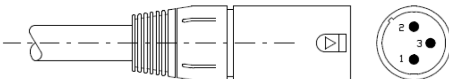
Afbeelding 1 XLR-stekker
