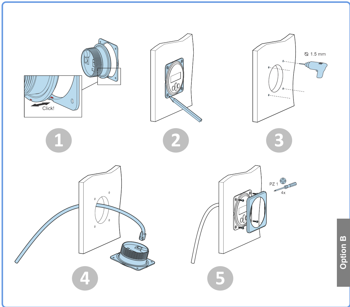
Befestigungsmöglichkeit B
