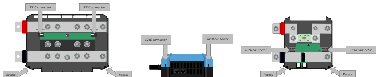
Placering av RJ10-kontaktidon och RJ10-kabelinfällningar på Lynx Distributor och Lynx Shunt VE.Can
