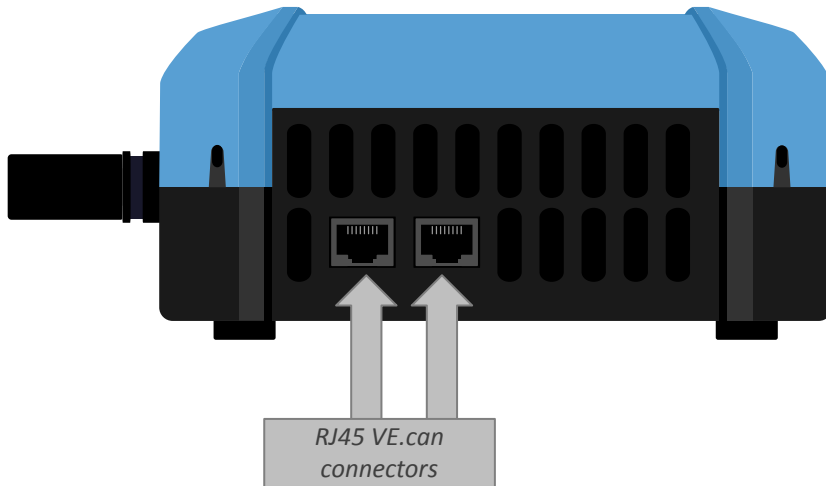
Placering av VE.Can-kontakt don Lynx Shunt VE.Can
