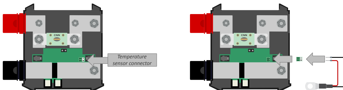
Temperatursensorsanslutning Lynx Shunt VE.Can
