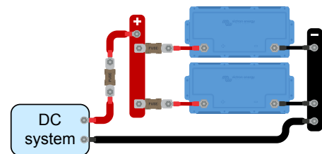
Mehrere Batterien parallel
