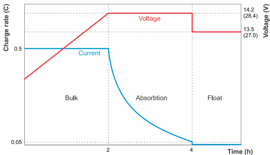
Laddningstabell litiumbatteri
