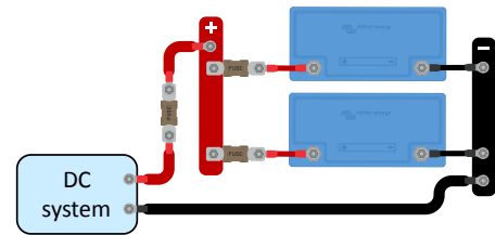
Flera batterier parallellkopplade
