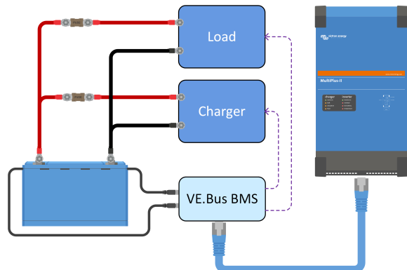
Het VE.Bus BMS V2 schakelt belastingen en laders uit via de "Load Disconnect" en bestuurt de omvormer/lader.
