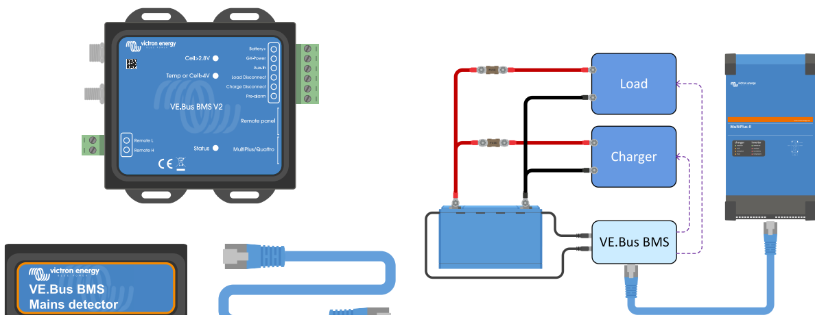
Le VE.Bus BMS éteint les consommateurs et les chargeurs avec « déconnexion de consommateur » et « déconnexion de chargeur », et contrôle le convertisseur/chargeur
