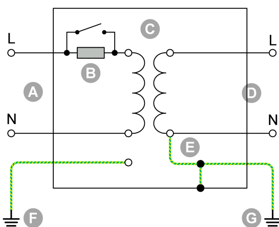
Esquema elétrico interno do transformador de isolamento.
