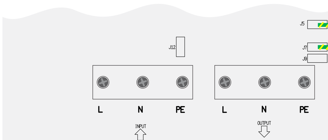
Neutralne wyjście AC (N) do uziemienia (PE).
