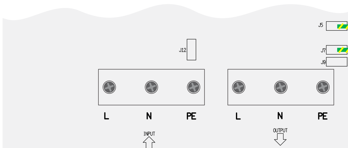
Saída CA neutra (N) para a ligação de terra (PE).
