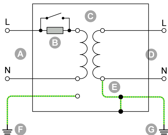
Isolationstransformatorns interna kopplingsschema.
