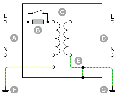
Schemat okablowania wewnętrznego transformatora separacyjnego.
