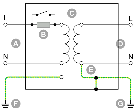
Schema di cablaggio interno del trasformatore di isolamento.
