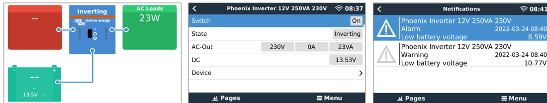
Приклад екранів GX зліва направо: екран системи, екран інвертора та повідомлення про тривогу.
