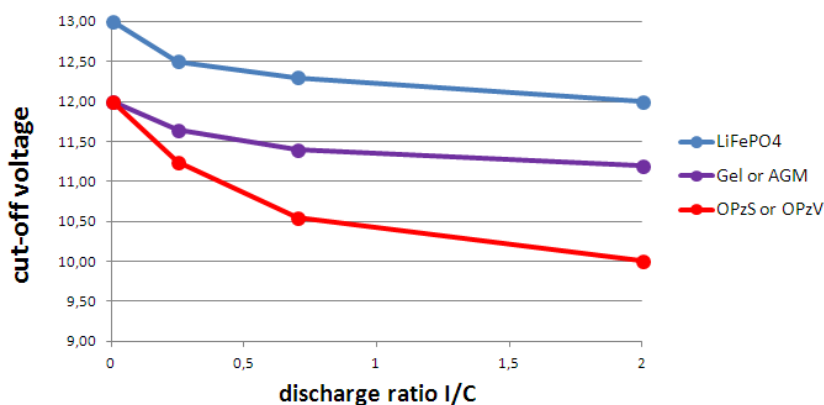
Графік співвідношення розряду та напруги батареї для різних типів батарей
