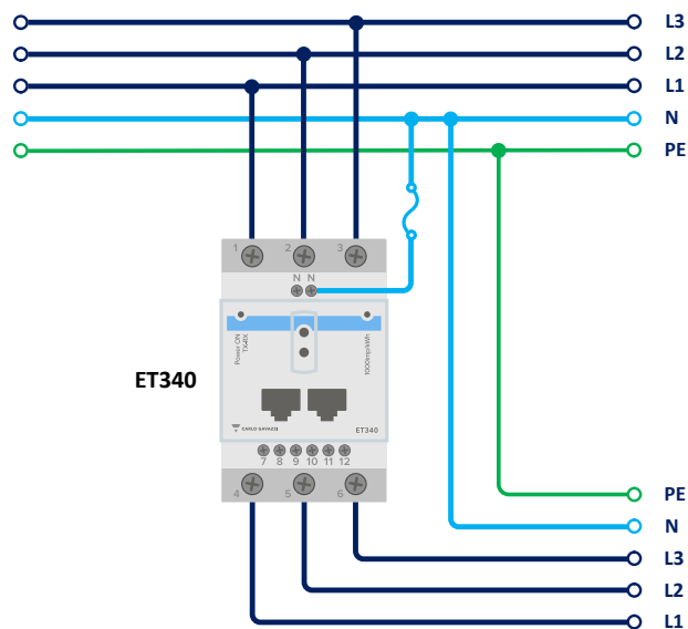
Cableado trifásico
