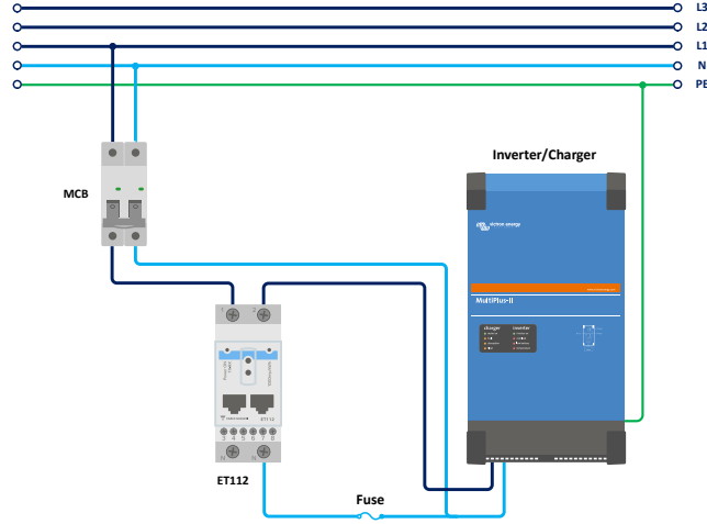
Şebeke Sayacı - Cihaz şebeke sayacı olarak kullanıldığında gerçekleşen kablo bağlantısı
