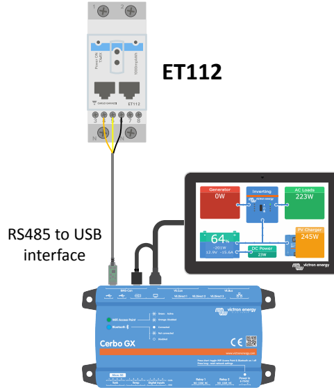
RS485 – USB arabirimi kullanılarak Cerbo GX cihazına yapılan kablolu ET112 bağlantısı
