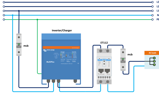
AC Sayacı - Cihaz bir İnvertördeki/Şarj Cihazındaki AC çıkışını ölçmek için kullanıldığında gerçekleşen kablo bağlantısı
