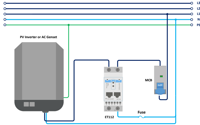
PV İnvörtör - Cihaz PV invertörü veya AC jeneratörü ölçmek için kullanıldığında gerçekleşen kablo bağlantısı
