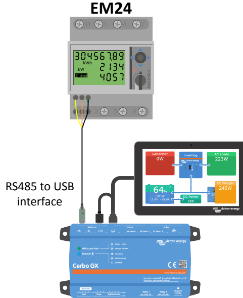
RS485 – USB arabirimi kullanılarak Cerbo GX cihazına yapılan kablolu EM24 bağlantısı
