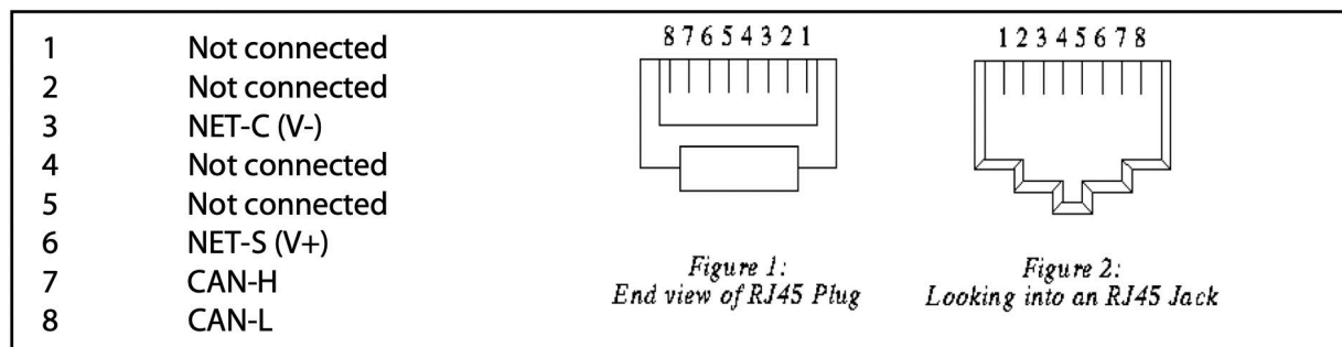
Victron VE.Can-penbezetting
