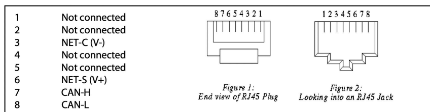
Pinos de saída Victron VE.Can
