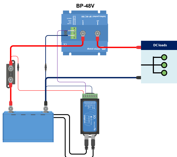
BatteryProtect folosește deconectarea consumatorului unui smallBMS
