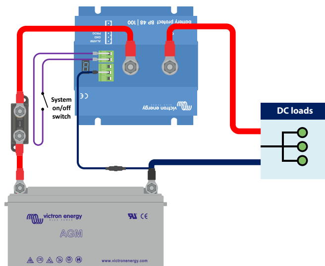
BatteryProtect cu comutator pornit/oprit de la distanță
