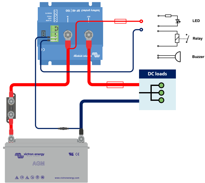
Conectarea unui LED, a soneriei sau a releului la ieșirea BatteryProtect
