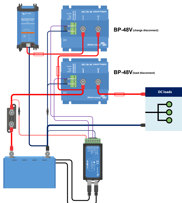
Două BatteryProtect preiau controlul asupra unui încărcător și a unui circuit de sarcină
