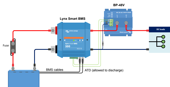
BatteryProtect în modul Li-ion controlat de ATD de la un Lynx Smart BMS
