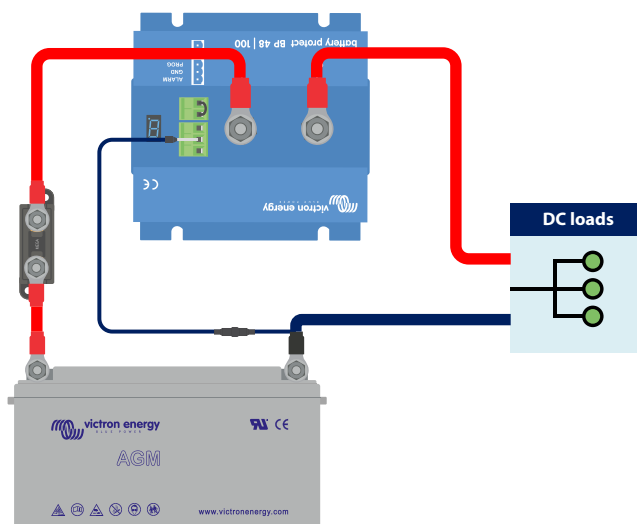
BatteryProtect dans un système simple avec une boucle de fil entre les deux broches du connecteur de la borne distante (réglage d'usine)
