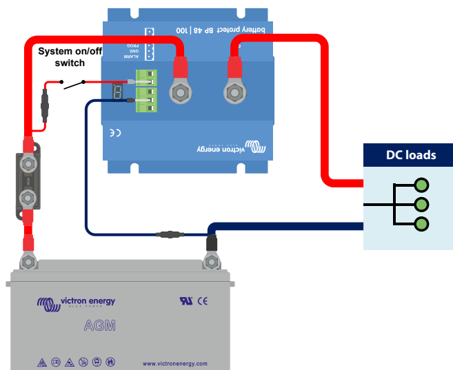
Interrupteur câblé entre le positif de la batterie et la broche REMOTE de la borne distante
