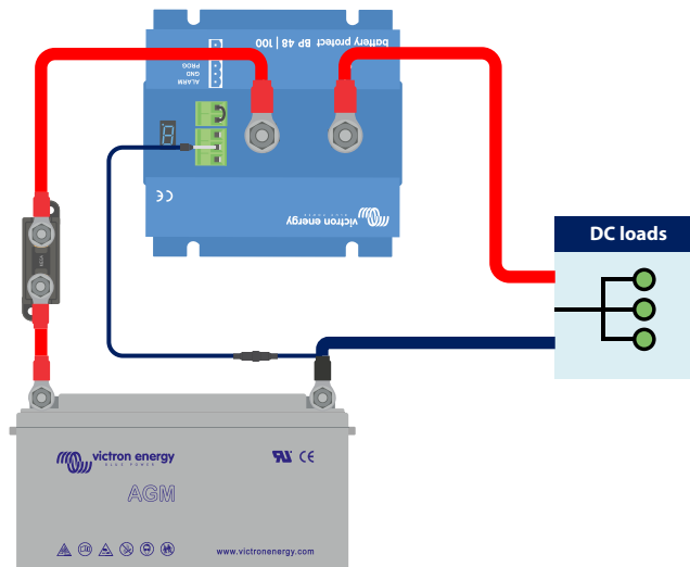
BatteryProtect en un sistema sencillo con anilla metálica entre los dos pines del conector terminal remoto (predeterminado de fábrica)
