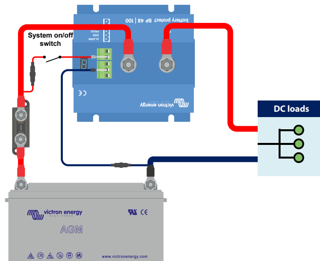
Interruptor conectado entre el positivo de la batería y pin REMOTE del terminal remoto
