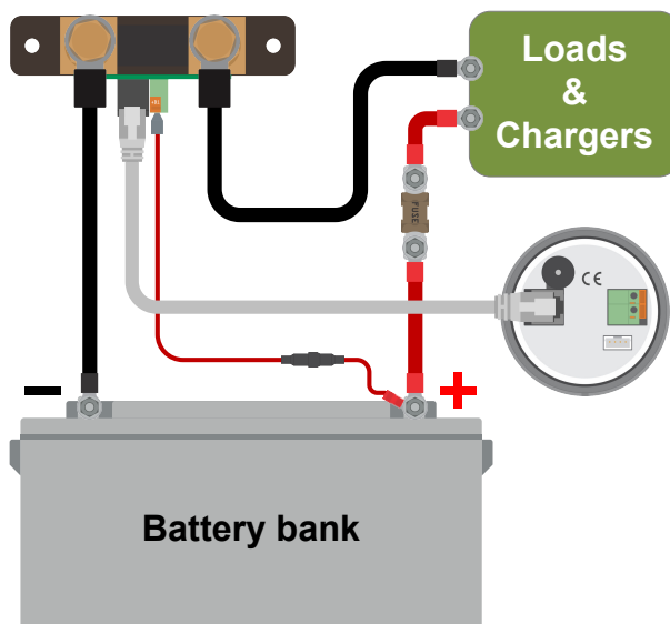
Grundläggande installation av batteriövervakare.
