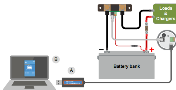
Exempel över en VE.Direct till USB-gränssnittsanslutning mellan batteriövervakaren och en dator.
