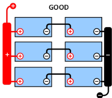
GOOD (bine): Punctele mediane nu sunt conectate; sunt utilizate bare de interconectare, dar fără monitorizarea punctului median.
