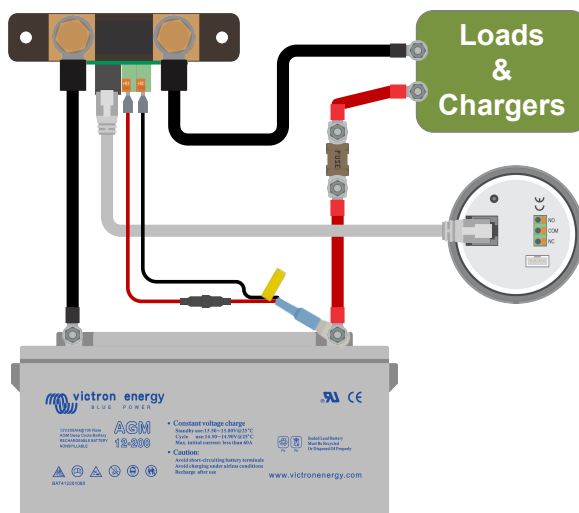
Sistem de monitorizare a bateriei cu sistem de detectare a temperaturii auxiliar.
