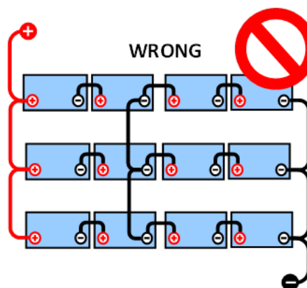
WRONG (greșit): Punctele mediane sunt conectate și nu există bare de interconectare sau monitorizare a punctului median.
