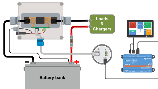
De accubewaker is verbonden met een Cerbo GX en een GX Touch scherm.
