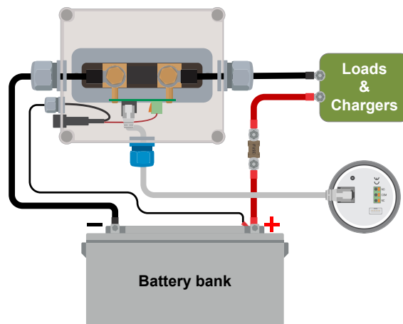
Installatie basis accubewaker.
