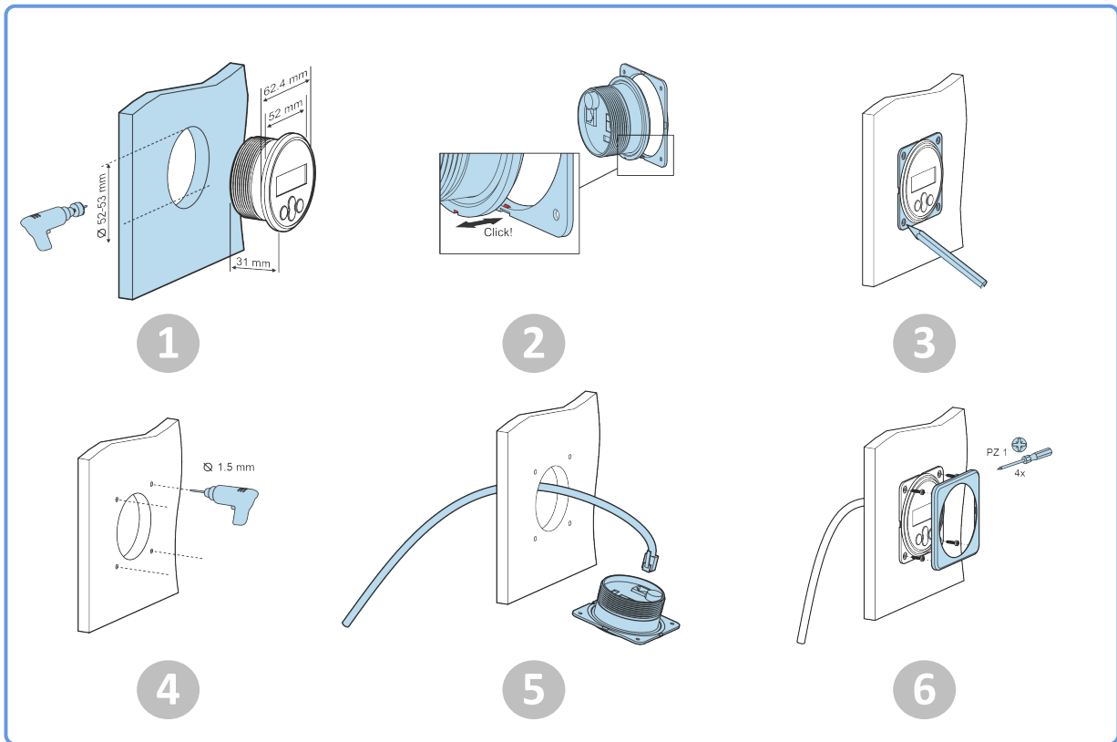
Monteringsmetod B.
