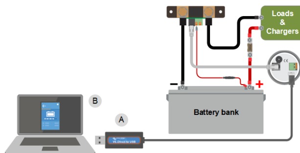
Exemplu de conexiune a unei interfețe VE.Direct to USB între sistemul de monitorizare a bateriei și un computer.
