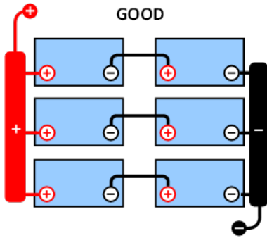
GOOD (correto): Os pontos médios não estão conectados; os barramentos são utilizados, mas sem monitorização do ponto médio.
