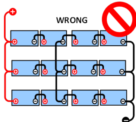
WRONG (incorreto): Os pontos médios estão conectados e sem barramentos ou monitorização do ponto médio.
