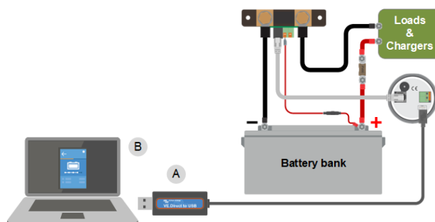
Exemplo de uma ligação de «interface» VE.Direct para USB entre o monitor de bateria e um computador.
