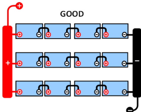
GOOD (correto): Os pontos médios não estão conectados; os barramentos são utilizados e sem monitorização do ponto médio.
