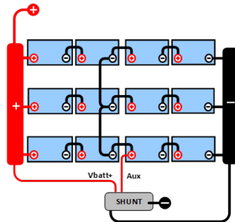
GOOD (correto): Os pontos médios estão conectados, os barramentos são utilizados e com monitorização do ponto médio.
