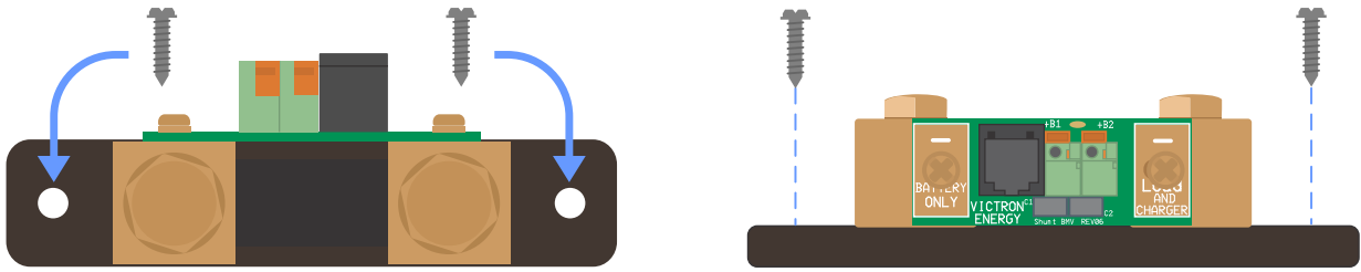
Vista superior do derivador «shunt» que indica os orifícios de montagem e vista lateral do derivador «shunt» que indica o método de montagem.
