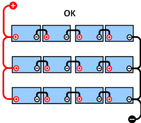
GOOD (correto): Os pontos médios não estão conectados e sem barramentos ou monitorização do ponto médio.
