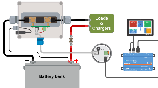
Batteriövervakaren är ansluten till en Cerbo GX och en GX Touch-skärm .
