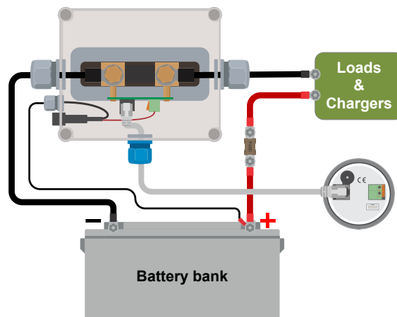
Installation de base du contrôleur de batterie.
