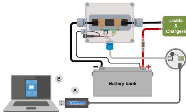
Exemple de branchement d'une interface VE.Direct-USB entre le contrôleur de batterie et un ordinateur.
