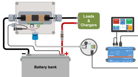
Der Batteriemonitor ist mit einem Cerbo GX und einem GX Touchscreen verbunden.
